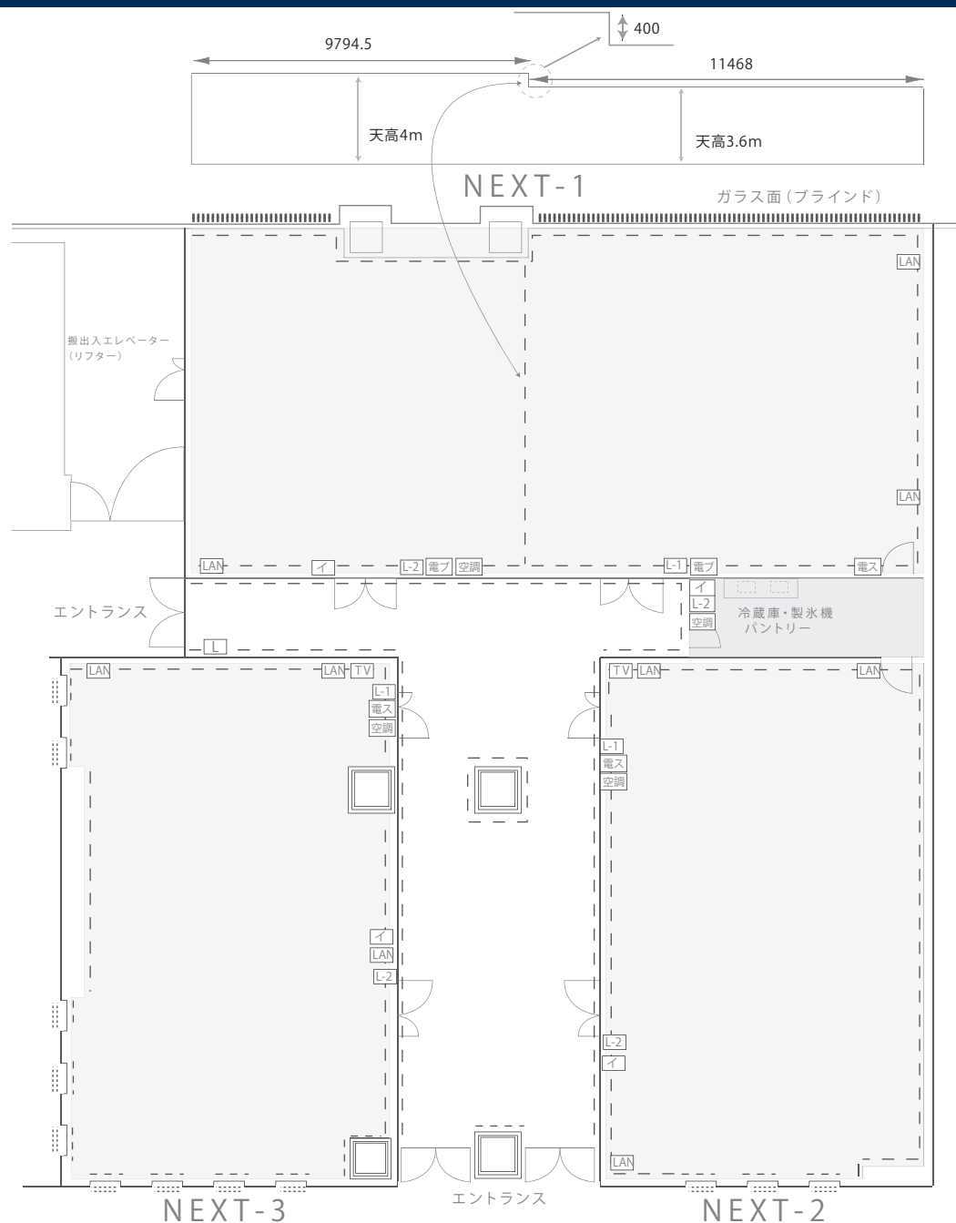
縮尺: 1/200 (A4)
